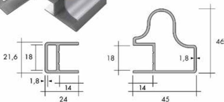
verstevigingsprofiel
